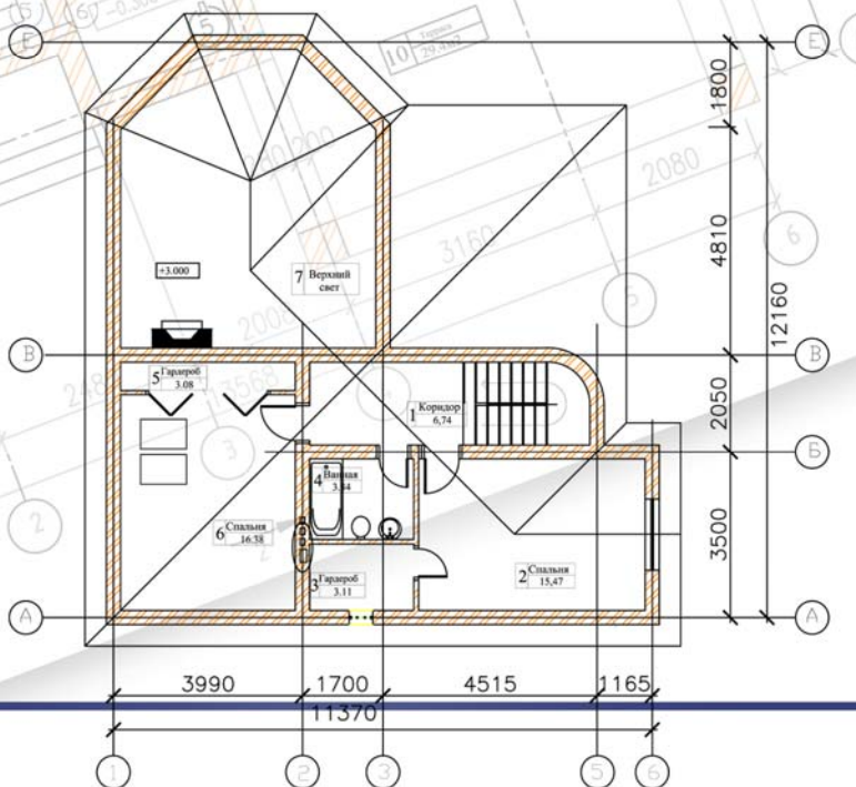
План 2 этажа S=48.62м 2
