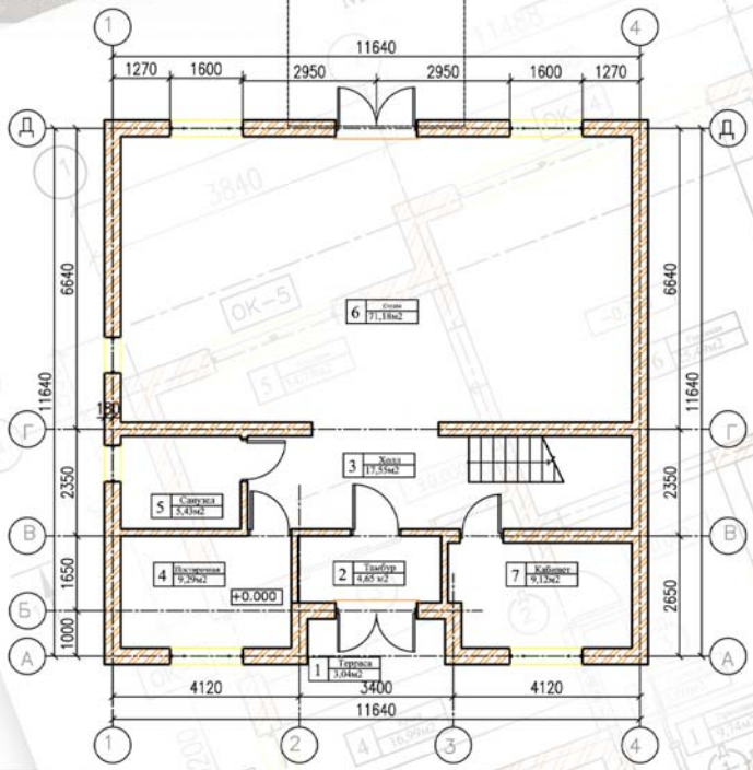
План 1 этажа S=120.93м2
