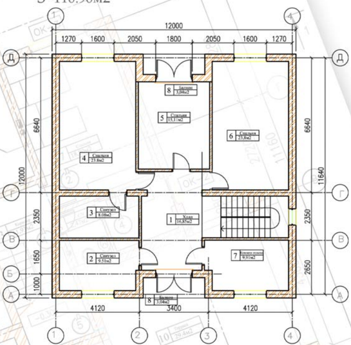
План 2 этажа S=110.90м2
