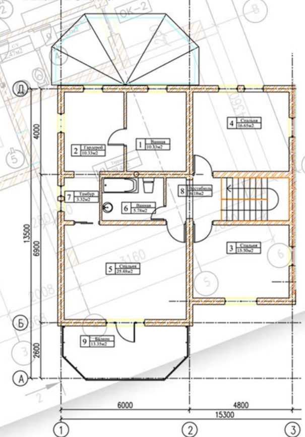
План 2 этажа
